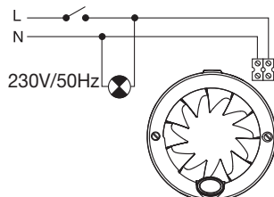
elektrické zapojení
