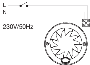
elektrické zapojení
