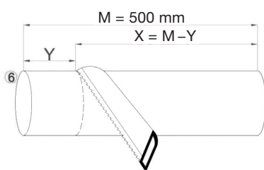
obr. 3.2 - zkrácení tubusu
