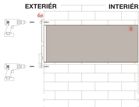
obr. 3.6 - vyvrtání otvorů pro šrouby
