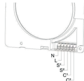
obr. 3.17 - zapojení svorkovnice
