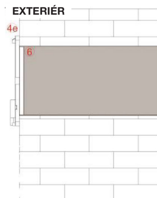
obr. 3.4 - montážní rámeček
