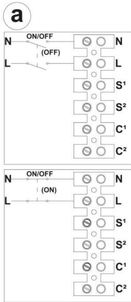
obr. 3.16 - zapojení nástěnného přepínače
