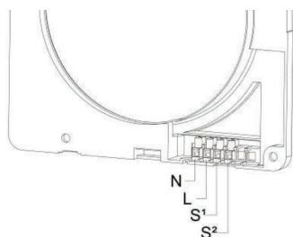
obr. 3.14 - připojení RESPIRO 150
