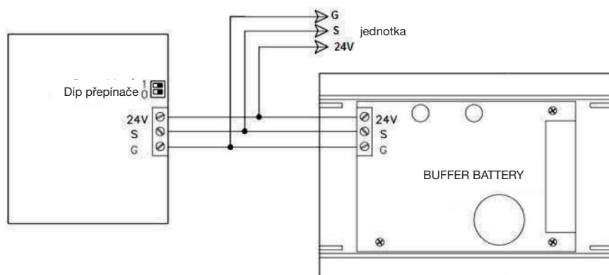
COP/CAV zapojení
